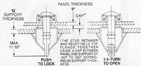
STUD SPLIT RETAINER
