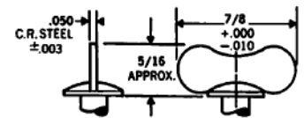
WING HEAD AW35 STUD TYPE 3
